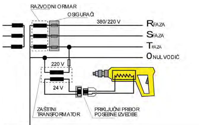
Sl. 6. Ručni električni alat priključen na maleni sigurnosni napon od 24 V izmjenične struje tzv. trošilo klase III.
